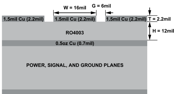
図 21. PCB 層構成例
