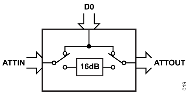
図 19. 簡素化した回路図
