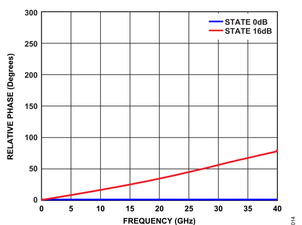
図 14. 全状態でのリアクティブ・フェーズと周波数の関係
