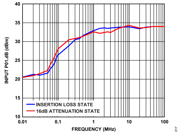
図 17. 入力 P0.1dB と周波数の関係、低周波数領域の詳細
