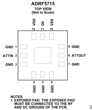
図 4. ピン配置
