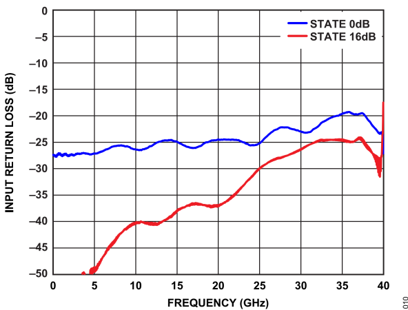
図 10. 全状態での入力リターン・ロスと周波数の関係
