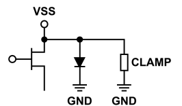
図 8. VSS のインターフェイス回路図
