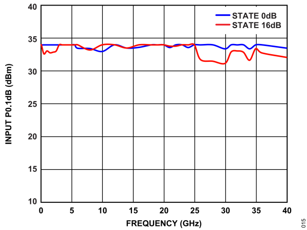
図 15. 入力 P0.1dB と周波数の関係
