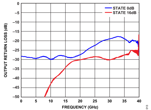
図 13. 全状態での出力リターン・ロスと周波数の関係
