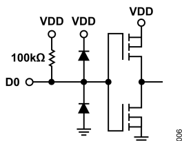
図 6. D0 のインターフェイス回路図
