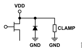
図 7. VDD のインターフェイス回路図
