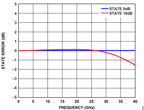
図 11. 全状態での状態誤差と周波数の関係
