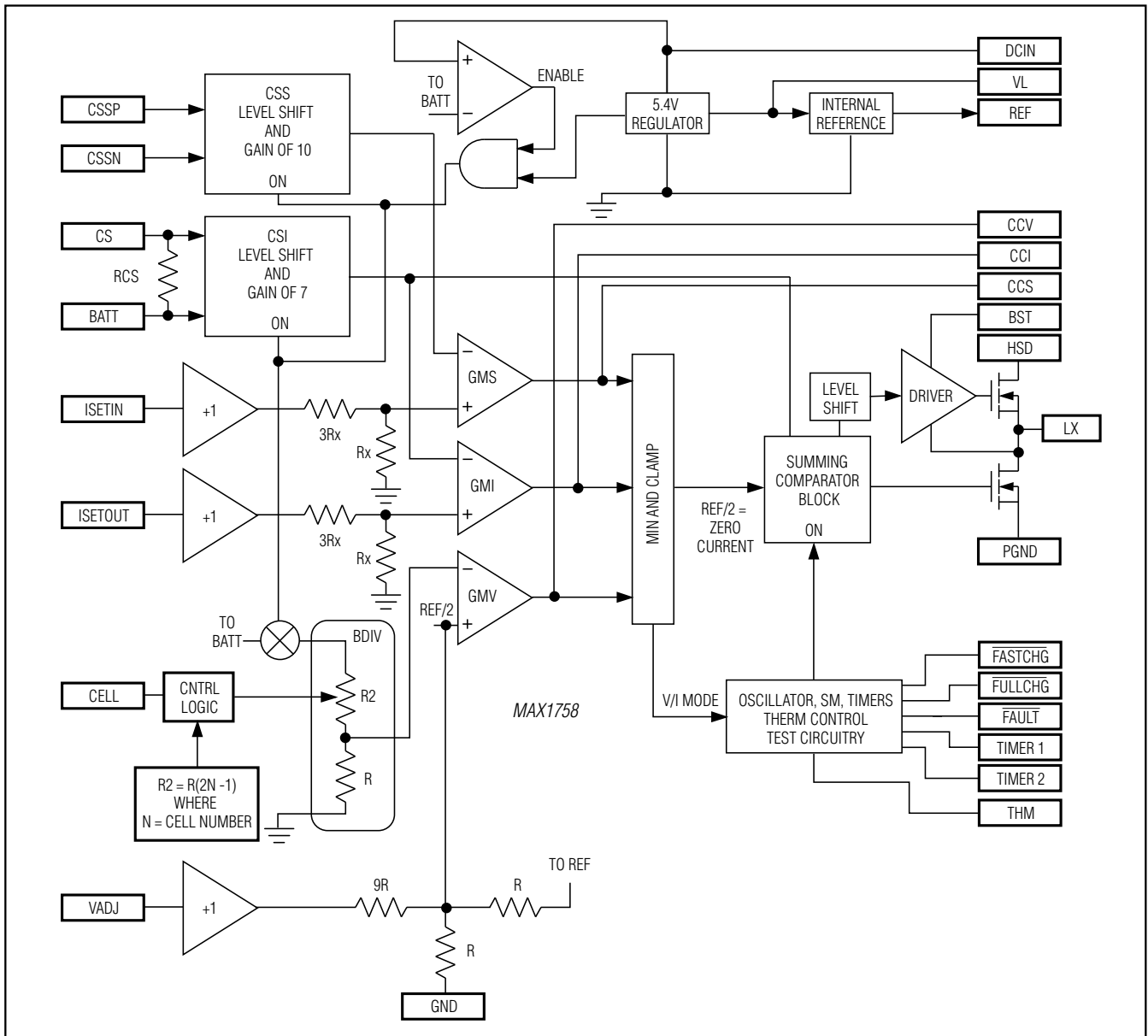
図3. MAX1758のファンクションダイアグラム
