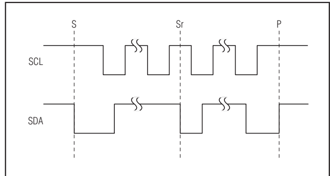
图7. START、STOP和REPEATED START条件
