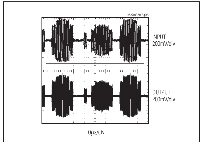
图5. MAX9670/MAX9671的色度(C)信号视频输出(图中所示为多发帧面图视频测试信号)
