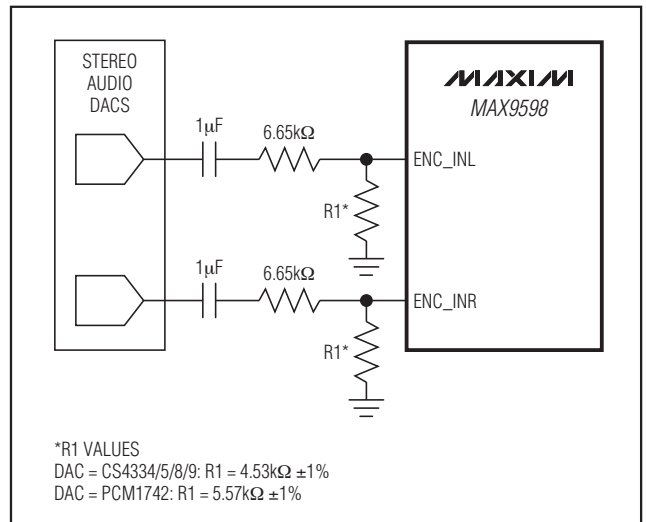
图13. 将音频源连接到音频输入的应用电路(1μF电容连接到以地为参考的电阻，将音频输入信号偏置到地电位，电阻用于衰减音频信号)
