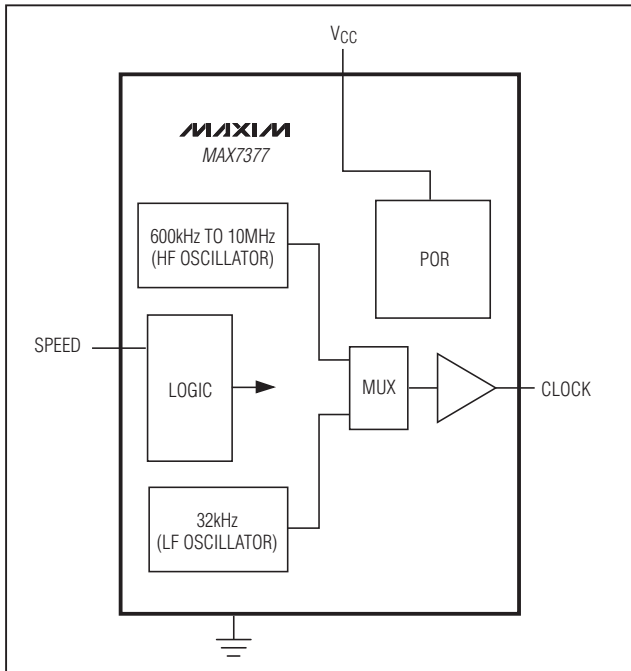
图1. 功能框图
