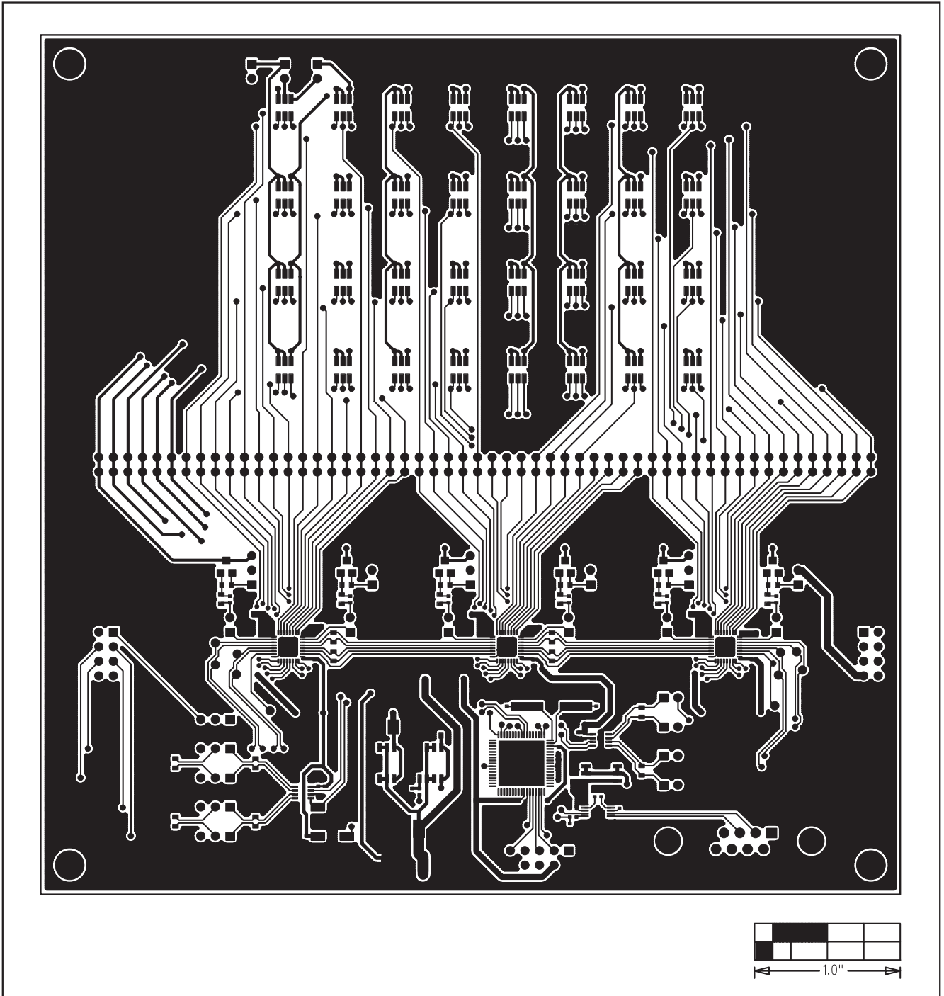
图7. MAX6972评估板PCB布局—元件层
