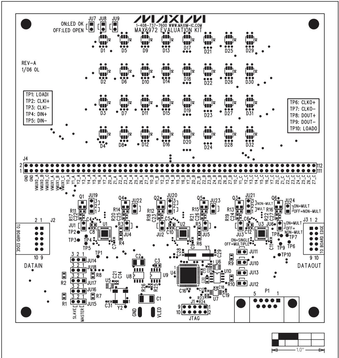
图6. MAX6972评估板PCB元件布局—元件层
