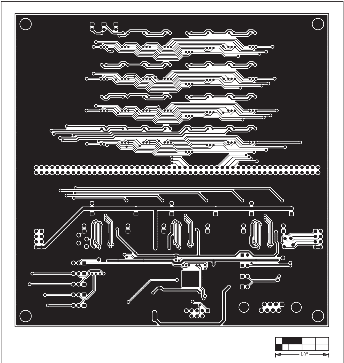
图8. MAX6972评估板PCB布局—焊接层
