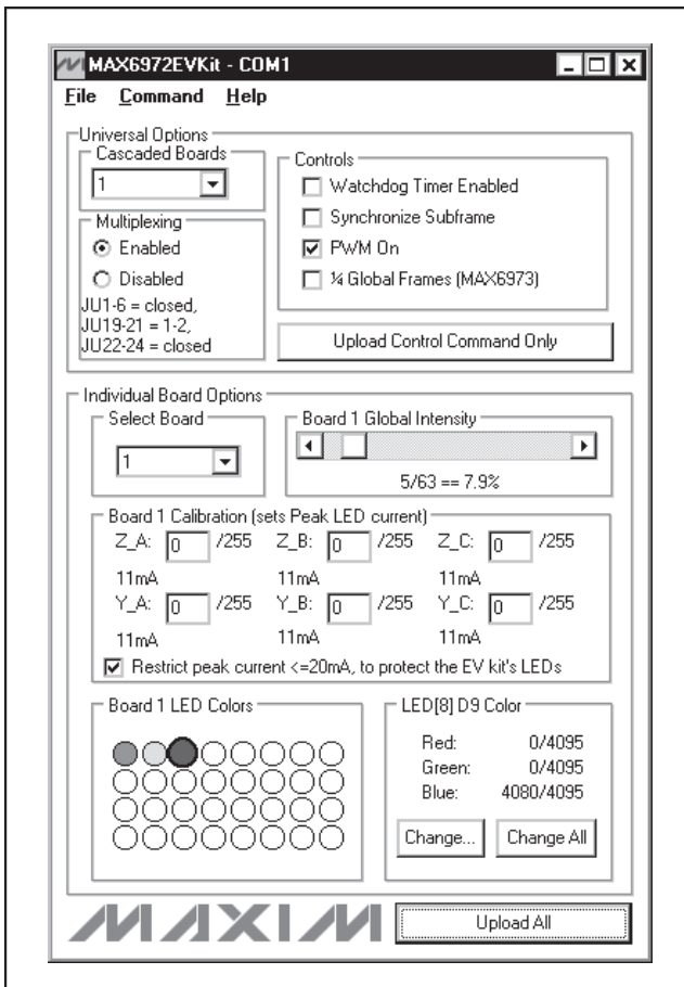
图2. MAX6972评估板—连接至COM1的主窗口
