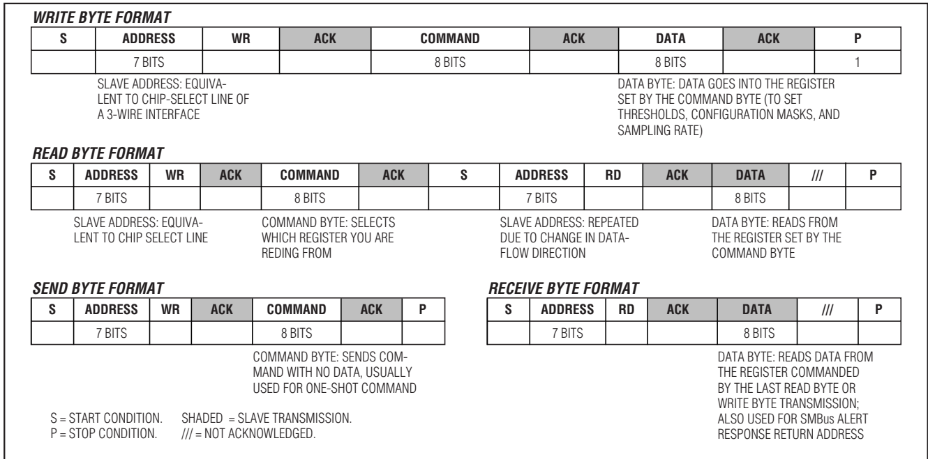
图2. SMBus总线协议
