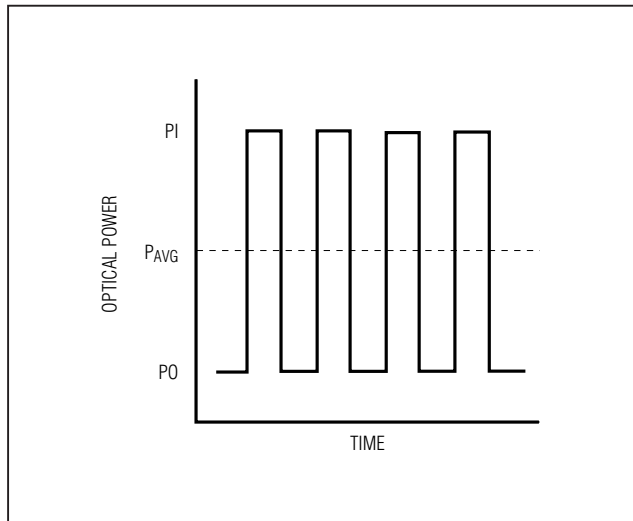
图6. 光功率关系
